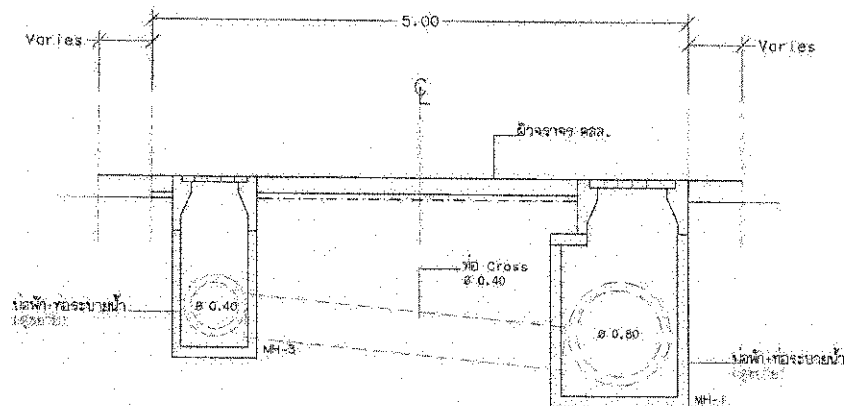
รูปตัด B-B มาตราส่วน 1:150
