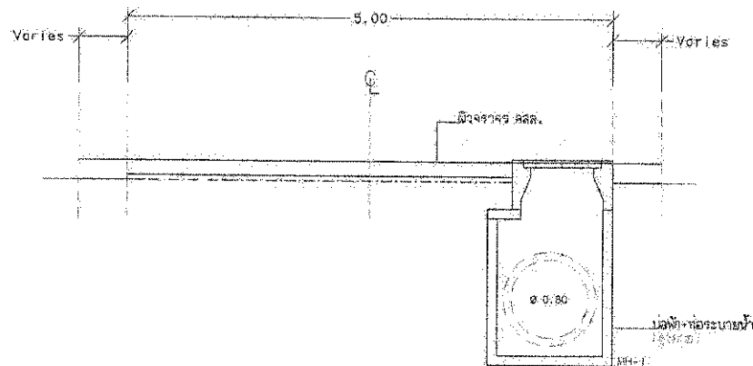
รูปตัด A-A มาตราส่วน 1:150
